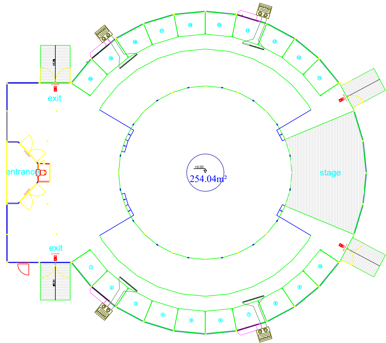
VUE EN PLAN CLIMATISATION AVEC 4 ROOFTOP
